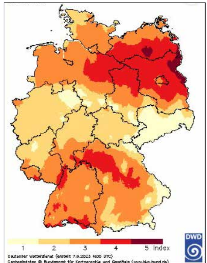
Waldbrandindex des DWD vom 07.06.2023
